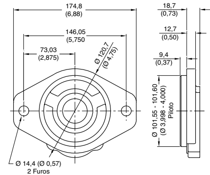
Flange SAE "B" de 2 furos (Código 97)
