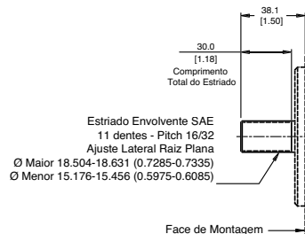
Estriado SAE 19-4 (Código 92)
